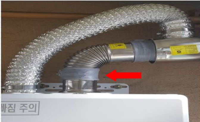
FF(강제급배기식)보일러
